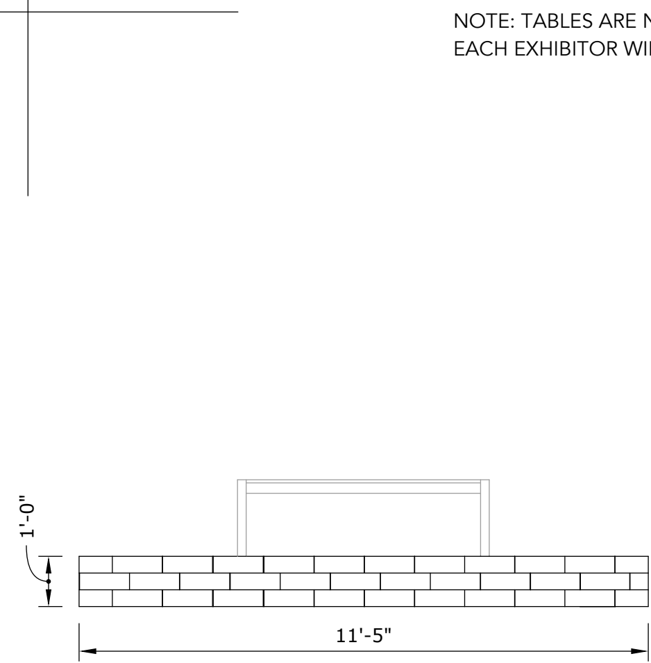
ELEVATION
